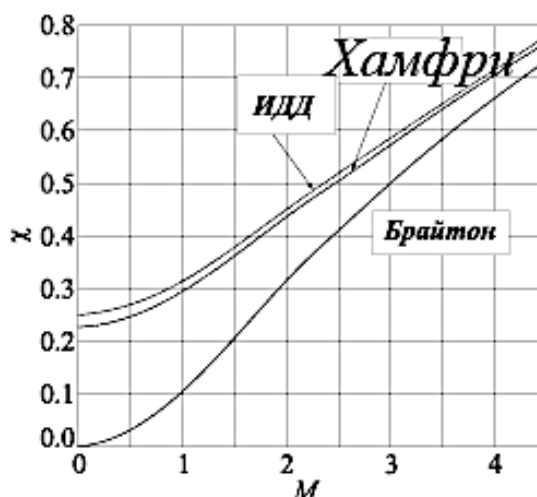
Рис. 8. Преимущество КПД термодинамического цикла проточного воздушно-реактивного (ПВРД) импульсно-детонационного двигателя (ИДД).
