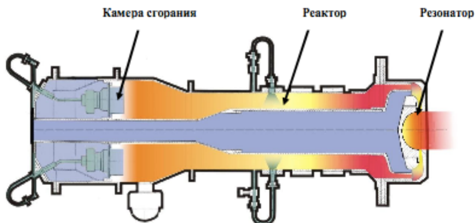
Рис. 13. Схема ИДД с высокочастотным резонатором.
