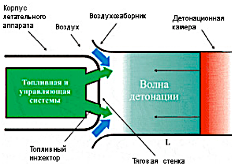
Рис. 11. Принципиальная схема импульсно-детонационного двигателя (ИДД).
